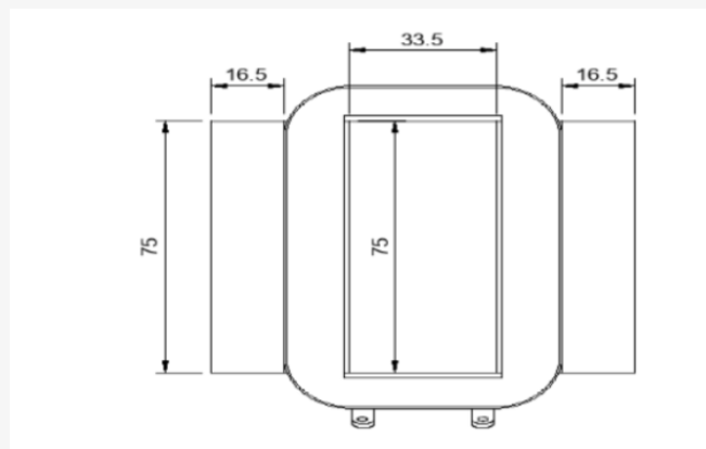
Figura 6. Perímetro teórico del bobinado (unitario)
