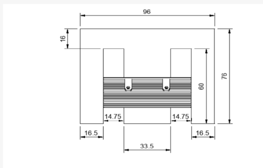
Figura 5. Especificaciones del Chapado (visto de frente)
