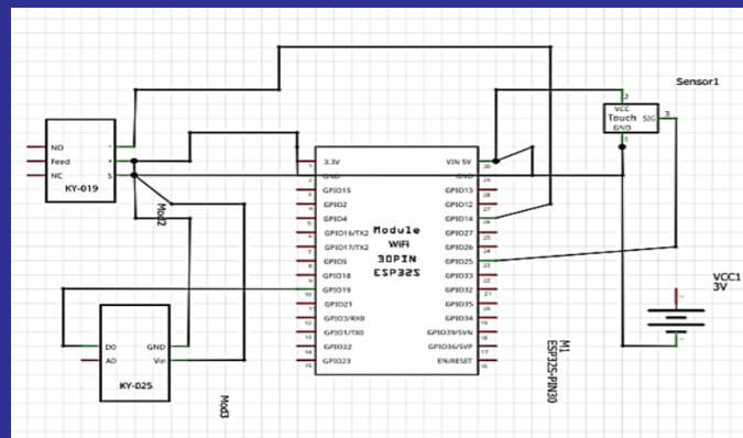
Figura 13. Esquemático de conexiones.
