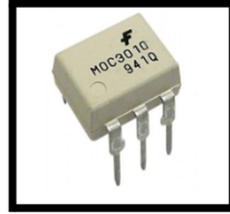
Figura SEQ Figura \* ARABIC 5 Optoacoplador Moc3010
